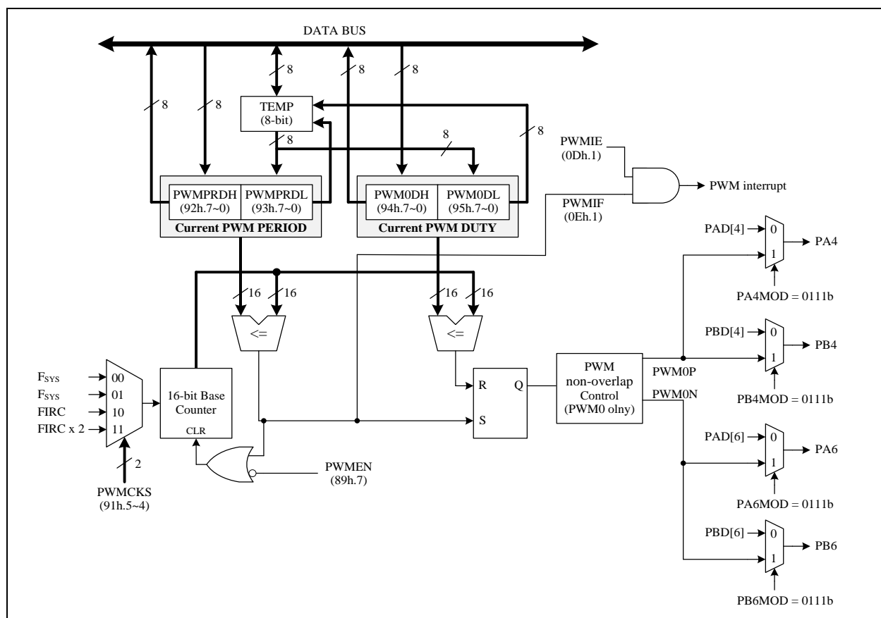
PWM0 框图
